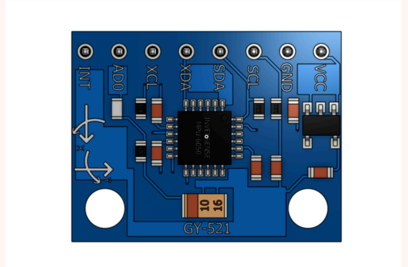
MPU 6050
